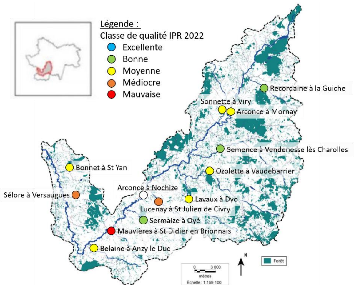
Figure 1 : Classe de qualité du peuplement piscicole par la note IPR pour chaque station étudiée dans le bassin de l'Arconce lors de l'année 2022.
