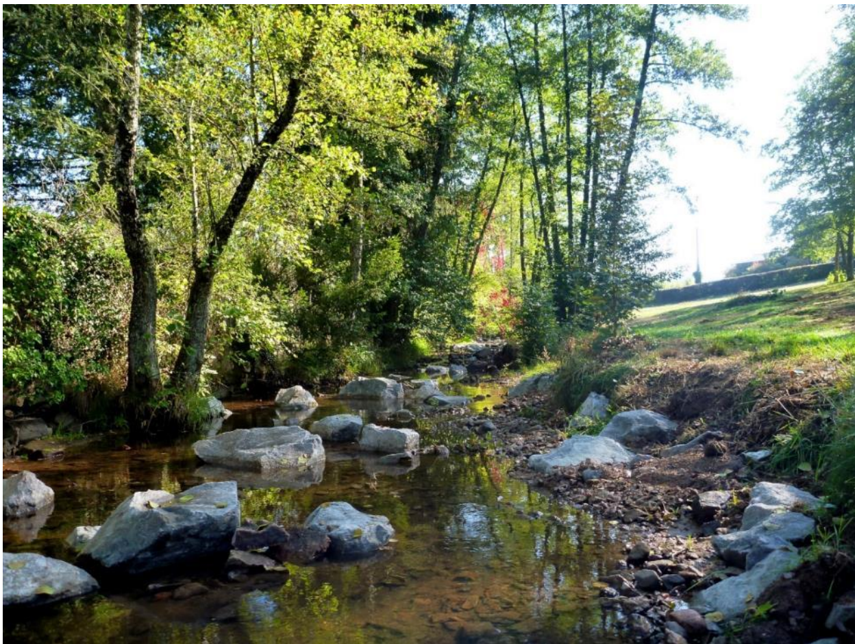
Blocs nouvellement posés dans le lit du Botoiret
