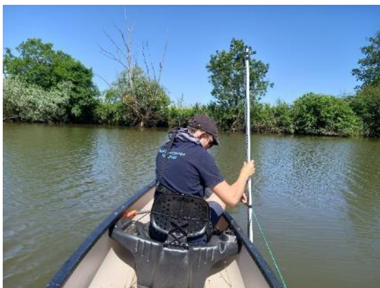
Relevé des hauteurs d'eau sur le bras mort de la Grande Seugnière
