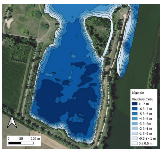
Carte bathymétrique de la partie sud de la gravière
